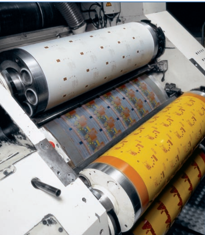
Печатен цилиндр за отпечатването на банкноти от 50 евро и гумено печатно платно в офсетова печатна машина
